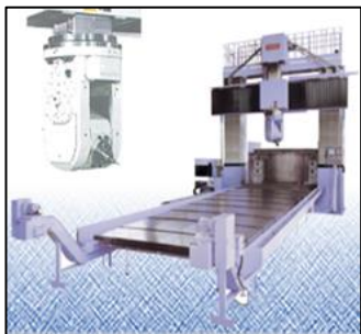
高速マルチセンタ(5面加工機・RB-4M II)
